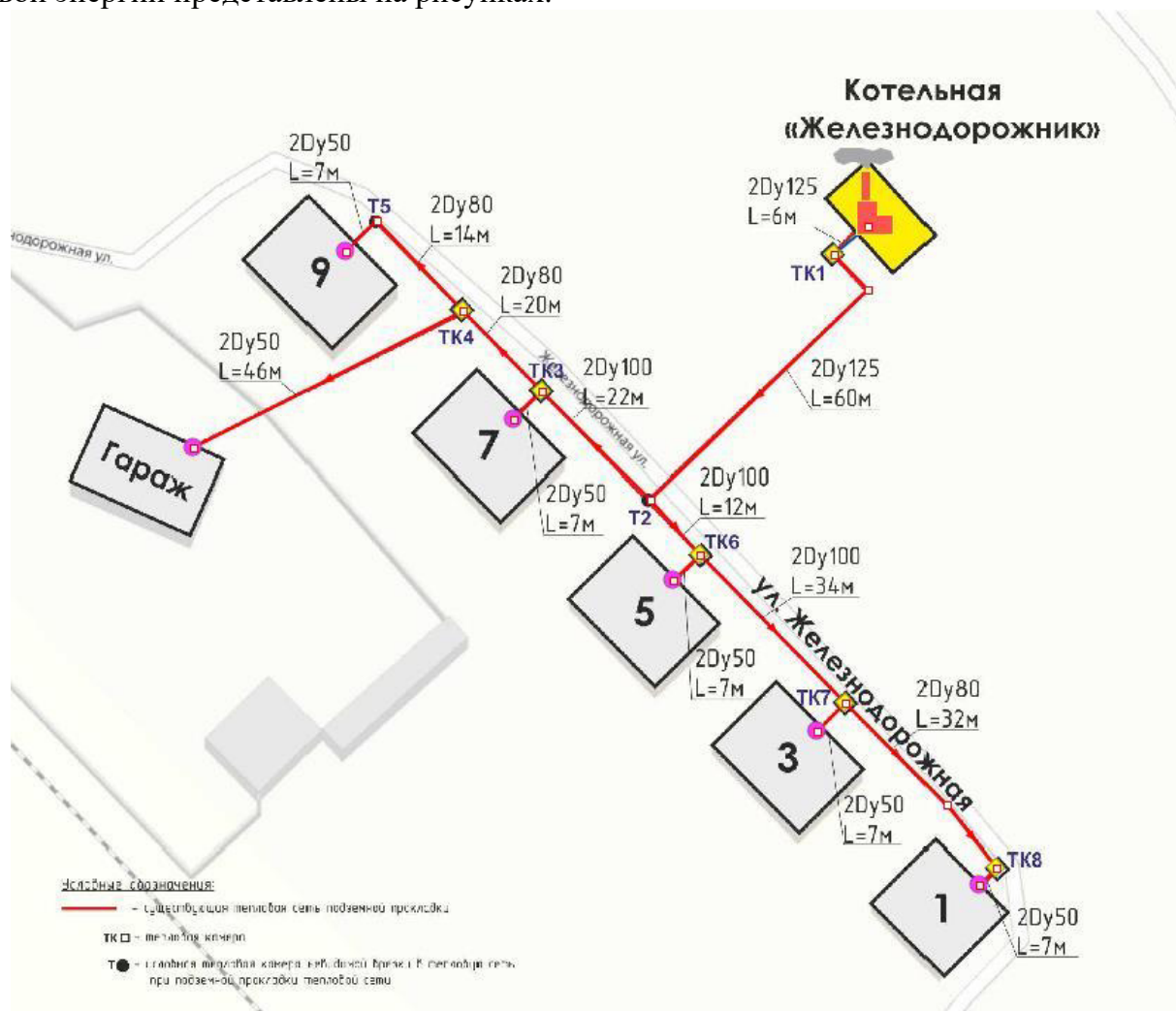
Рисунок 2 Схема теплоснабжения с. Кирба
