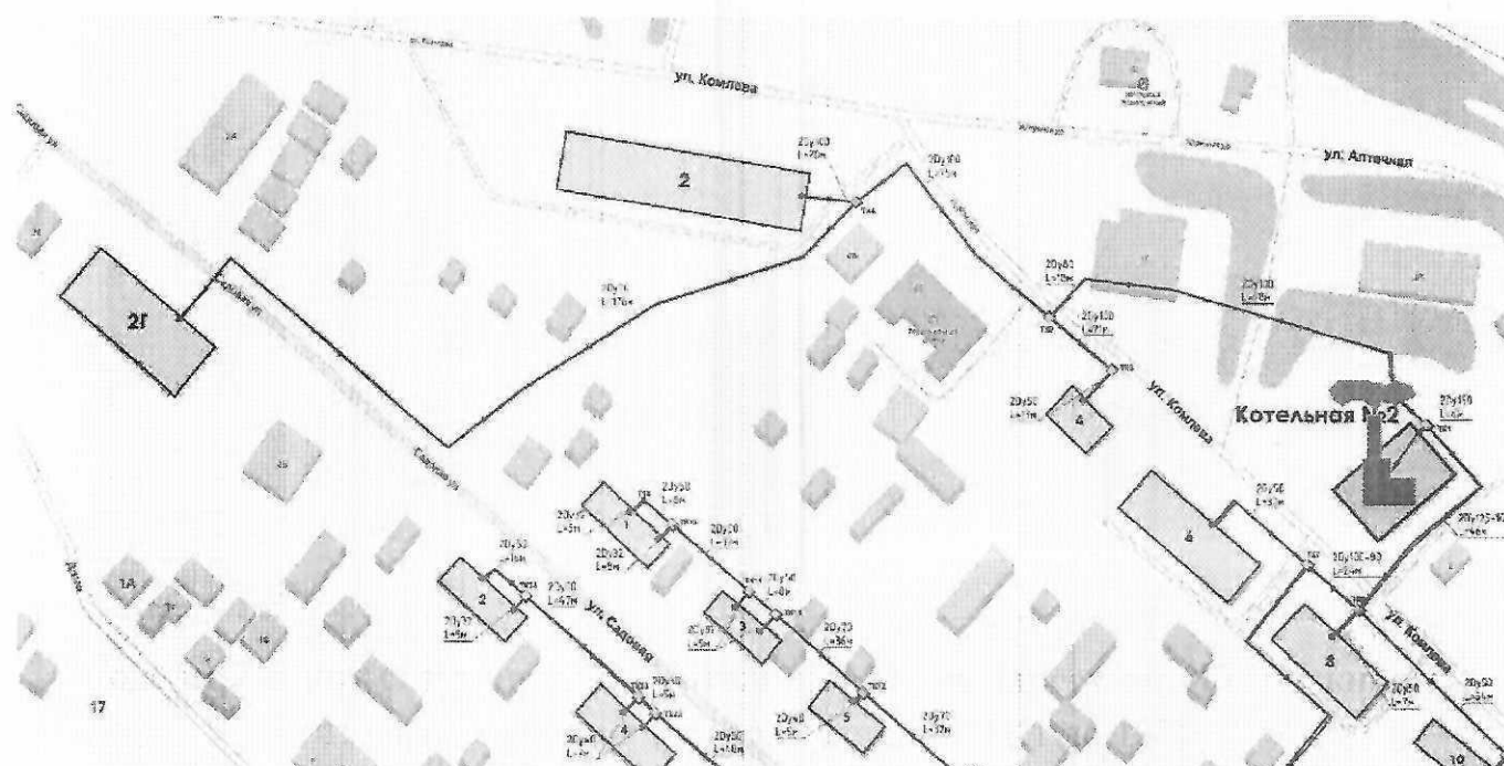
Рисунок 7.4.2. Визуализация отключения участка тепловой сети
