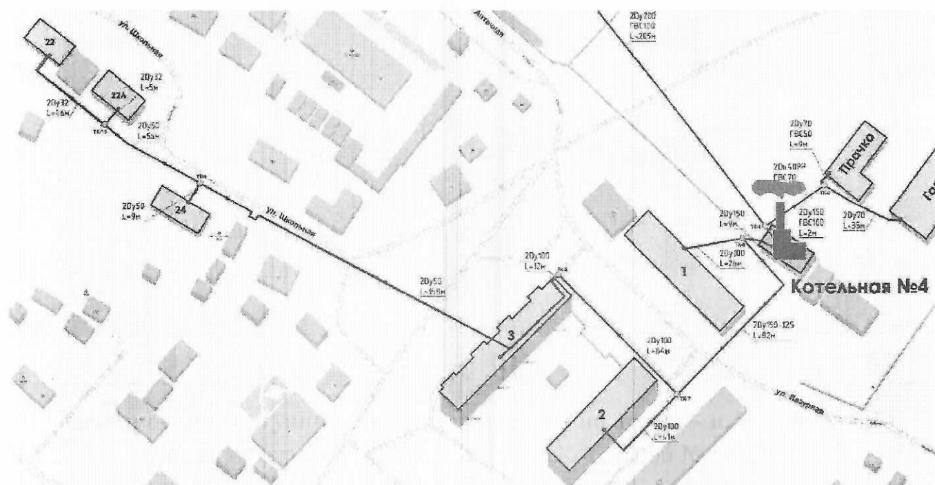
Рисунок 7.4.3. Визуализация отключения участка тепловой сети
