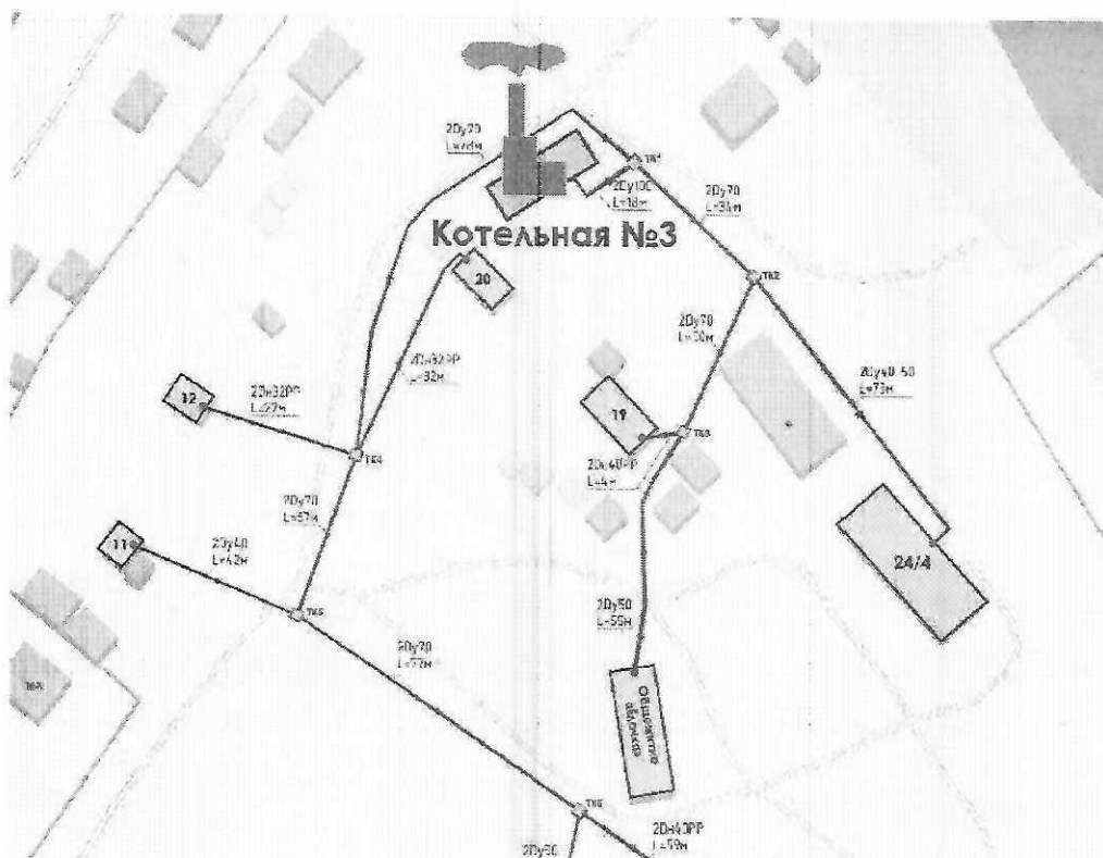
Рисунок 7.4.3. Визуализация отключения участка тепловой сети
