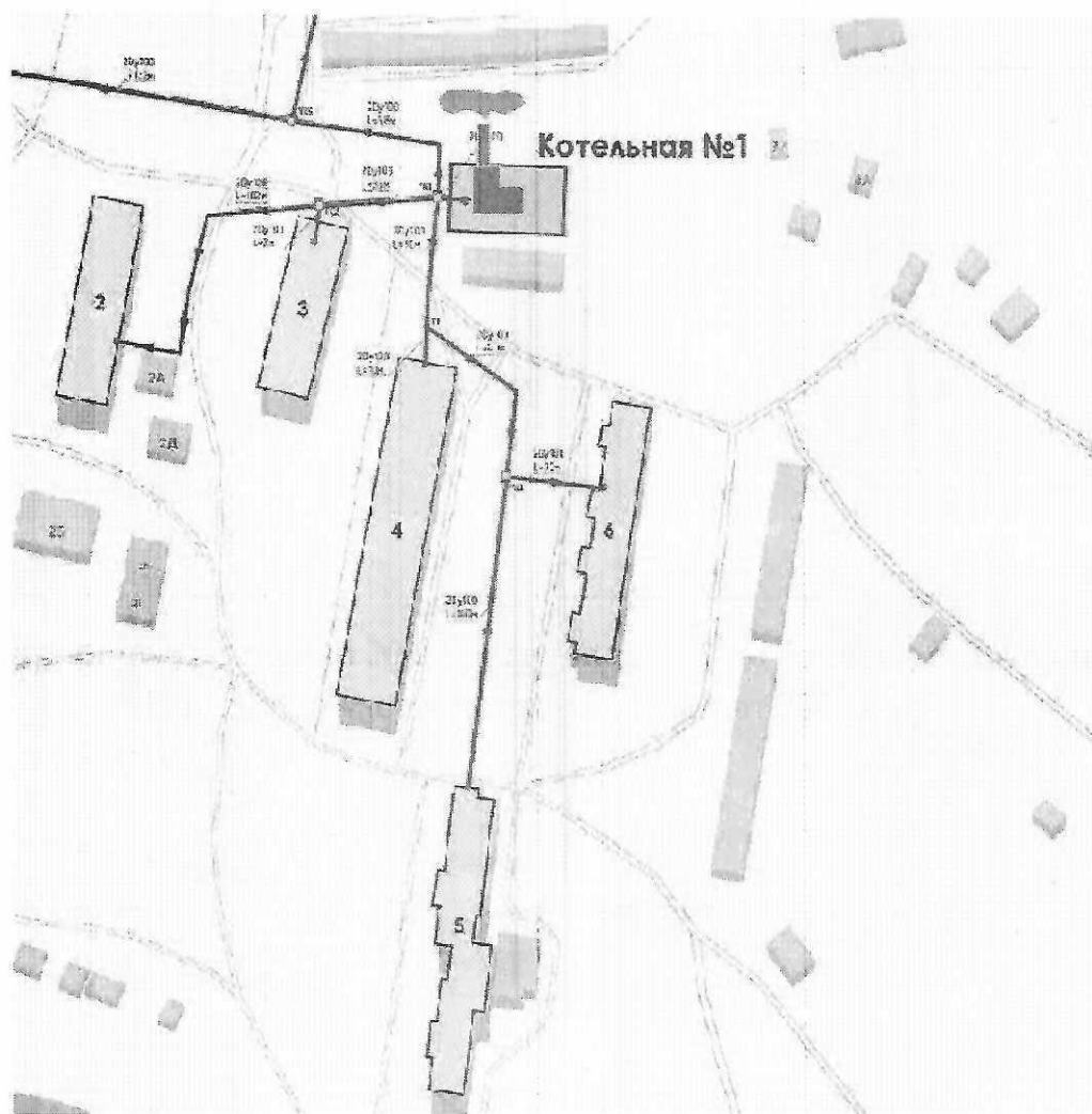
Рисунок 7.4.1. Визуализация отключения участка тепловой сети
