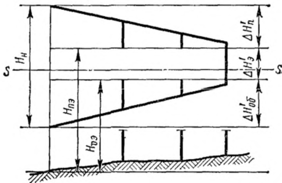
Рисунок 7 Пьезометрический график тепловой сети при пропорциональной разрегулировке абонентов.
