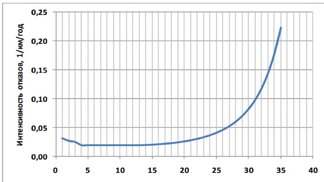
Рисунок 6 – Зависимость интенсивности отказов от срока эксплуатации участка ТС
